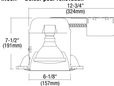
INC6R – Boîtier pour rénovation
