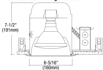
INC6 – Cadre de montage non isolé
