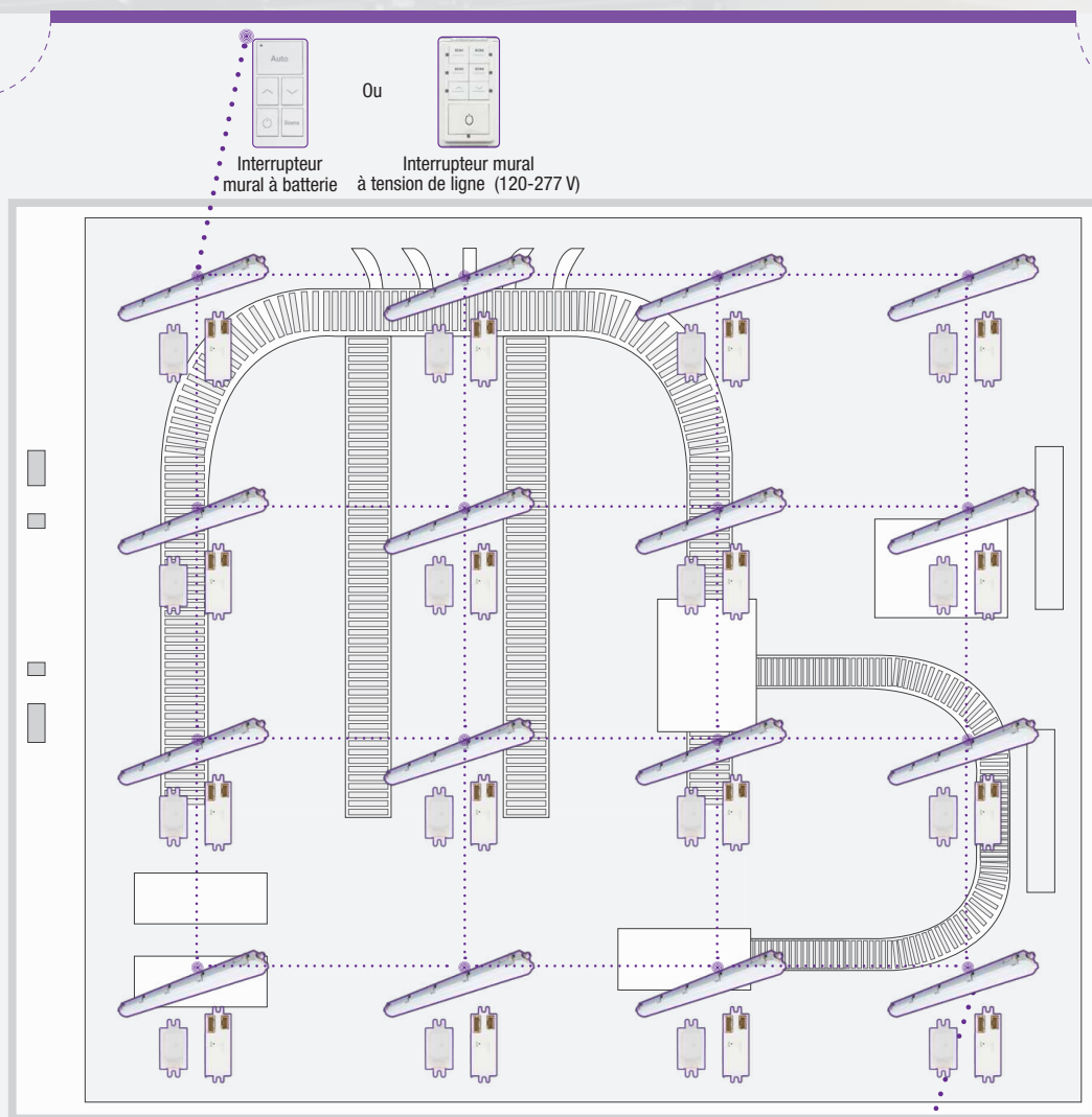
Usine de transformation alimentaire
