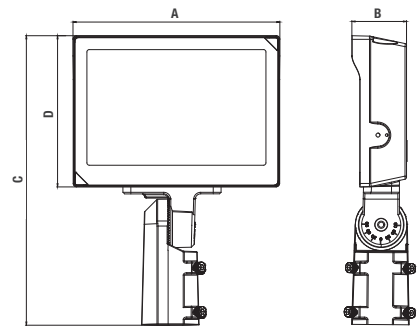
SLIPFITTER
