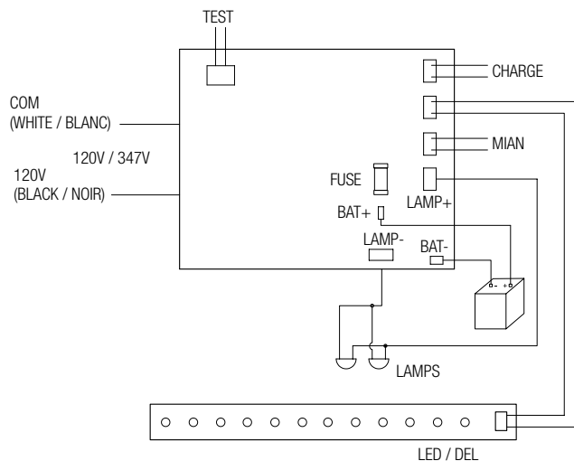
Fig. 3 Wiring diagram Schéma de câblage
