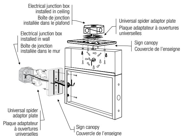
Fig. 4 Ceiling or end mount Montage au plafond ou par l'extrémité
