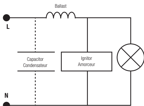
HPS/HID WIRING DIAGRAM SCHEMA DE CÂBLAGE SHP/DHI
